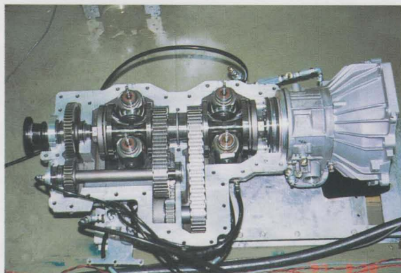
4 4輪駆動用トラクションドライブCVT
