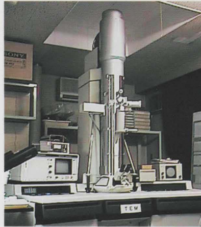
1 透過電子顕微鏡とAl合金中のクラック観察例
