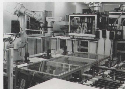
全自動製造工場でのロボットによる加工
